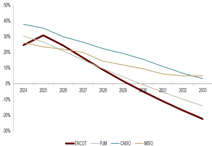
美國主要電網尖峰負載備用率
